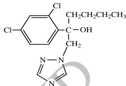
Hexaconazole (2-(2, 4-dichlorophenyl)-1-(2 H-1, 2, 4-triazole-1-Y1) hexan-2-O1)[C 14 H 17 Cl 2 N 3 O]
