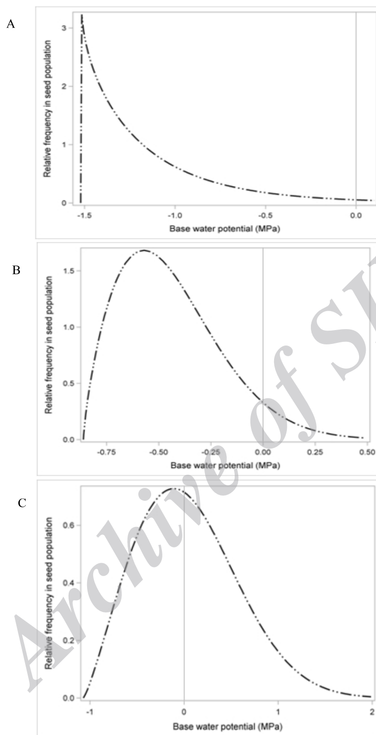
شکل ۶- تابع توزیع احتمال پتانسیل آب پایه پیش‌بینی شده با مدل هیدروتایم توسعه یافته بر مبنای توزیع ویبول برای
