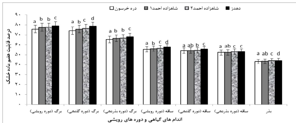
شکل ۳- درصد DMD اندام‌های برگ، ساقه و بذر گونه کنگر علوفه‌ای در رویشگاه‌های چهارگانه و سه مرحله فنولوژی
