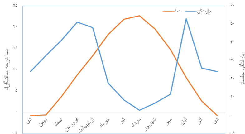
شکل ۲- منحنی آمبروترمیک ایستگاه آبجالوی سفلی در دوره آماری ۱۳۹۳-۱۳۴۵
