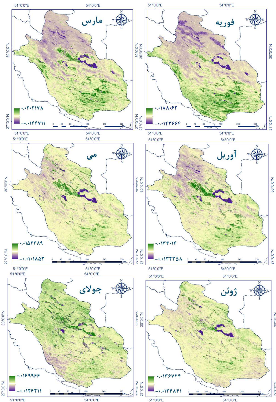
شکل ۲- نقشه‌ی تغییرات پوشش گیاهی با استفاده از آزمون تیل-سن
