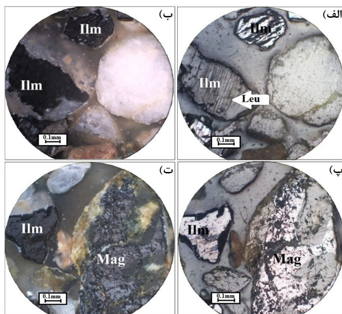
شکل ۷. تصویرهای میکروسکوپی بُرش‌های صیقلی تهیه شده از واحد پلاستی: الف و ب) ایلمنیت (Ilm) در حال دگرسان شدن به لوکوکسن (Leu)، پ و ت) همراهی ایلمنیت (Ilm) با مگنتیت (Mag) با بافت آواری (تصویرهای الف و پ در نور بازتابی PPL و تصویرهای ب و ت در نور بازتابی XPL)
