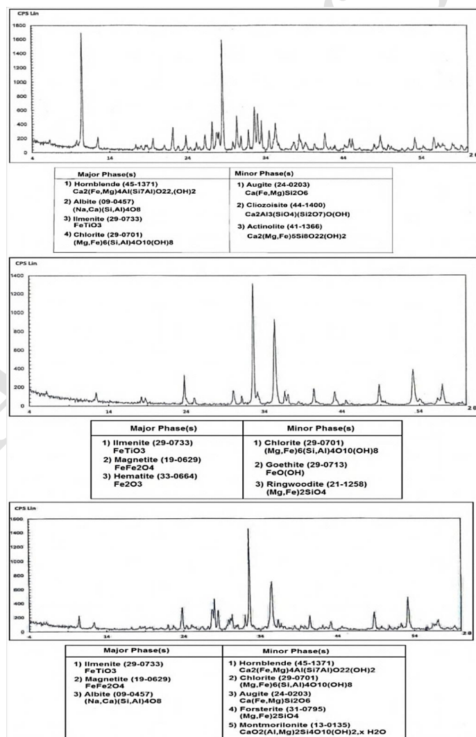
شکل ۸. نتایج آنالیز XRD نمونه‌های معرف پلاستر تیتان محدوده خانیک
