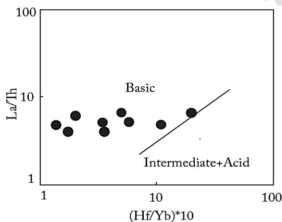
شکل ۱۴. جایگاه نمونه‌های پلاسر خانیک در نمودار دوتایی (Hf/Yb) \times 10 در برابر La/Th (هلاذیل و همکاران، ۲۰۰۳)
