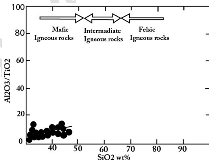
شکل ۱۲. پلات نمونه‌های رسوب پلاستیکی خائیک در نمودار Al_2O_3/TiO_2 در برابر SiO_2 (کالر، ۲۰۰۰)
