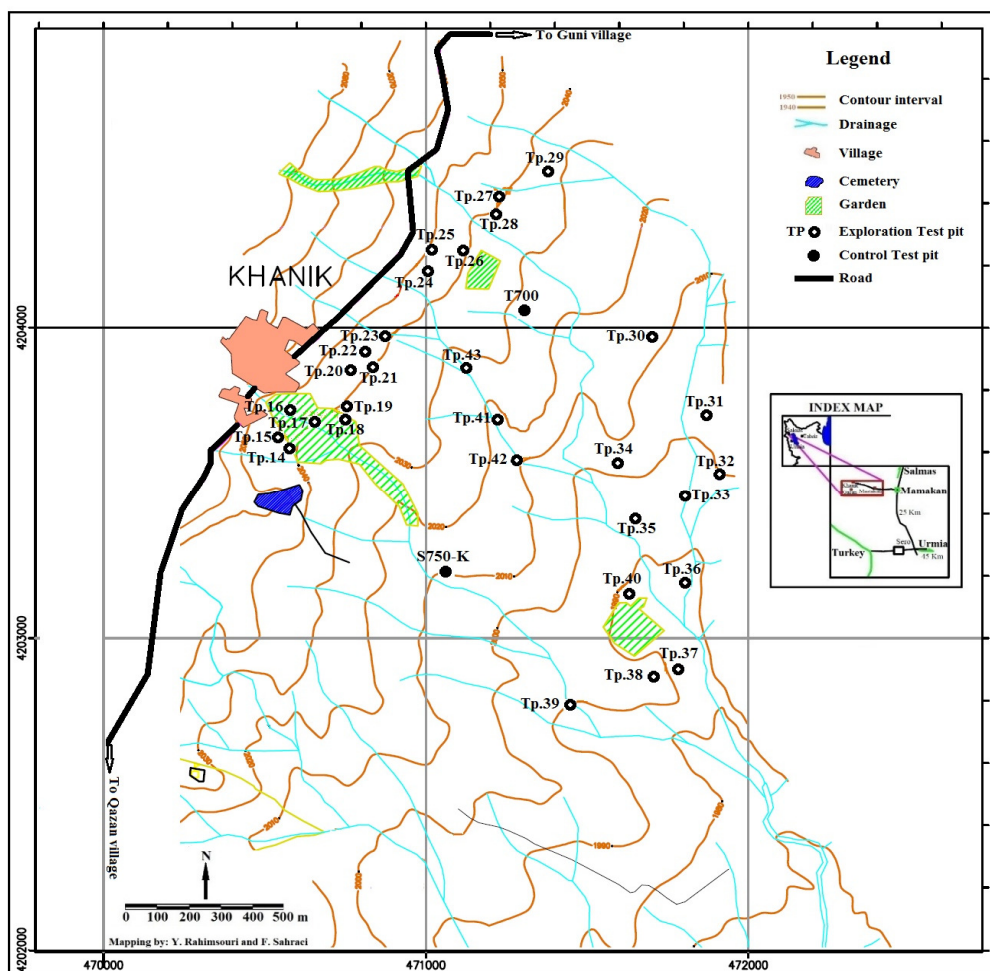
شکل ۳. جایگاه چاهک‌های اکتشافی محدوده تیتان پلاسری خانیک روی نقشه توپوگرافی با مقیاس ۱/۲۰۰۰۰
