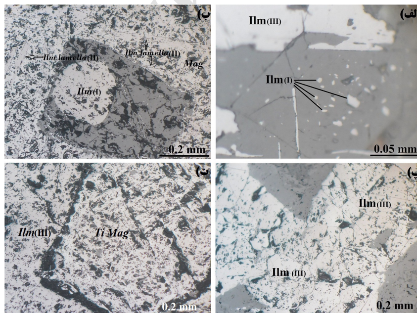
شکل ۶. تصویرهای میکروسکوپی نسل‌های مختلف کانی‌سازی ایلمنیت: الف) ایلمنیت نسل اول (I) بصورت ادخال درون باطله‌های سیلیکاته، ب) ایلمنیت نسل اول (I) بصورت ادخال درون باطله سیلیکاته و نسل دوم (II) بصورت تیغه‌هایی با بافت برون رست درون مگنتیت‌های نسل سوم، پ) ایلمنیت نسل سوم (III) با بافت دانه‌ای و پرکننده فضای خالی بین‌بلوری، ت) بلوری نیمه شکل‌دار از تیتانومگنتیت (TiMag) در همراهی با ایلمنیت نسل سوم (III).
