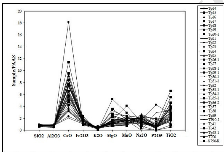
شکل ۱۱. الگوی توزیع عناصر اصلی رسوبات خائیک بهنجار شده نسبت به PAAS
