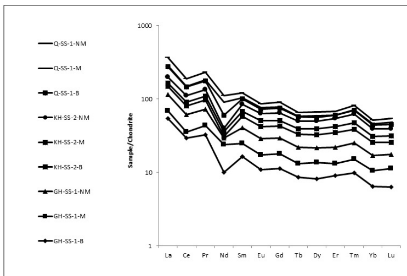
شکل ۱۳. الگوی توزیع REEs بهنجار شده به کندریت (تایلر و مک‌لینان، ۱۹۸۵) در نمونه رسوبات پلاسری منطقه خانیک
