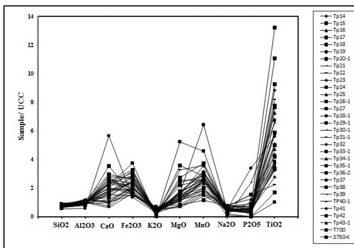
شکل ۱۰. الگوی توزیع عناصر اصلی رسوبات پلاستیکی خائیک بهنجار شده نسبت به UCC
