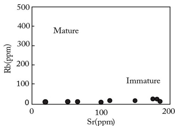
شکل ۱۵. جایگاه نمونه‌های پلاسما خانیک در نمودار Rb در مقابل Sr (پاتر، ۱۹۷۸)
