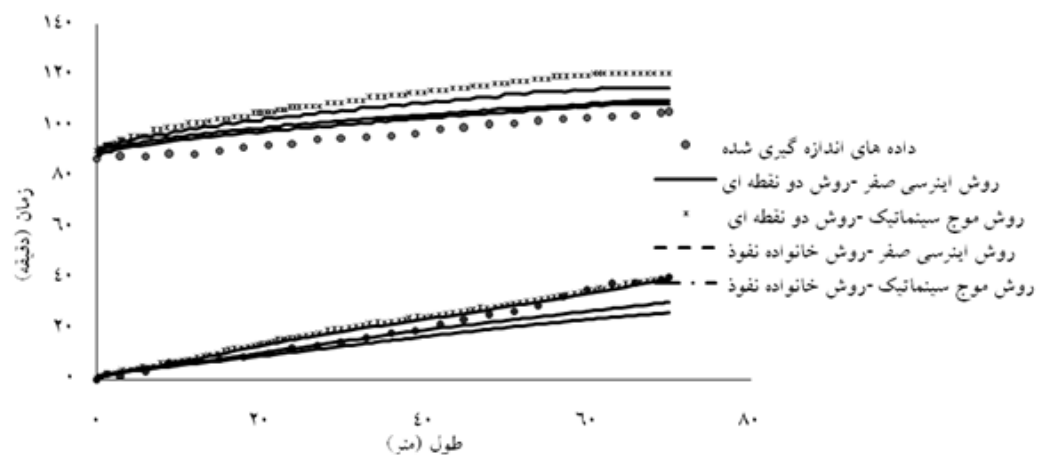
شکل ۶. منحنی‌های پیشروی و پسروی در حالت «ب» و مقایسه با داده‌های مزرعه‌ای
