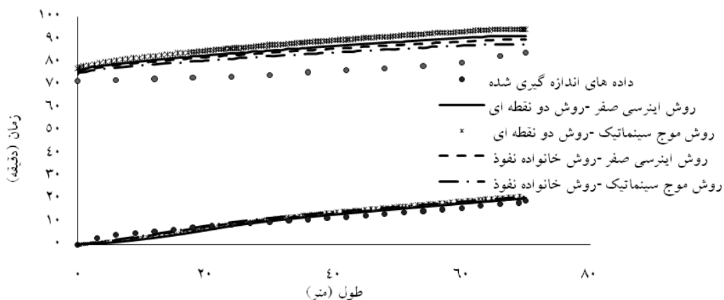
شکل ۷. منحنی‌های پیشروی و پسروی در حالت «ج» و مقایسه با داده‌های مزرعه‌ای
