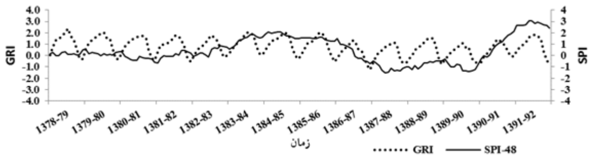
شکل ۶: نمودار تغییرات شاخص‌های GRI و SPI-48 در سفره تحت فشار
