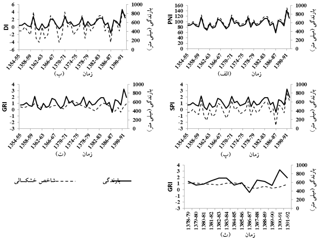
شکل ۴. نمودار تغییرات شاخص DI، PNI، SPI (الف، ب و پ) و GRI سفره آزاد (ت) و تحت فشار (ث) در برابر متوسط بارندگی سالانه
