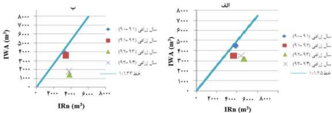
شکل ۳. نتایج ARIS شبکه آبیاری بالادست کانال یامچی (الف) و شبکه آبیاری قوریچای (ب)
