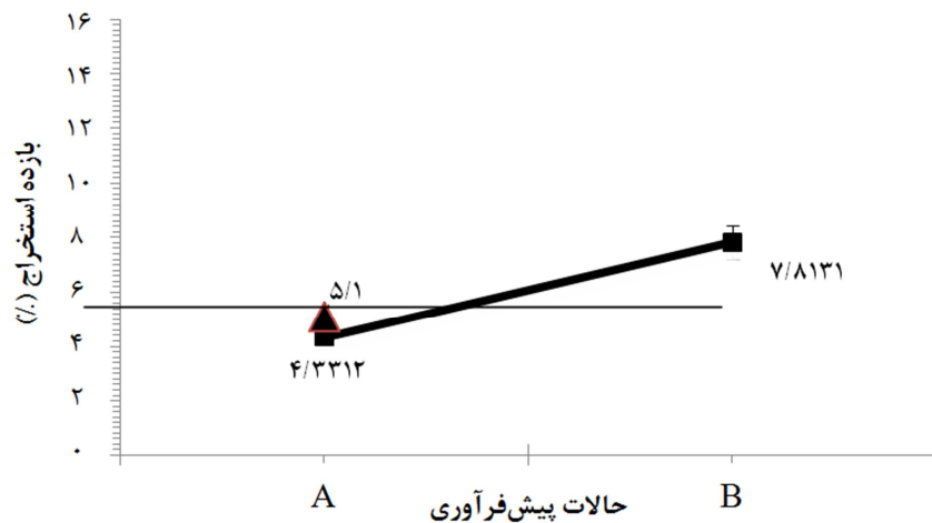
شکل ۱: بازده استخراج روغن از ریزجلبک Chlorella vulgaris . A: بدون پیش‌فرآوری. B: پیش‌فرآوری با آب گرم. نماد مثلث (▲) مشخص کننده میزان بازده در مطالعات گذشته است (Gouveia and Oliveira, 2009).
