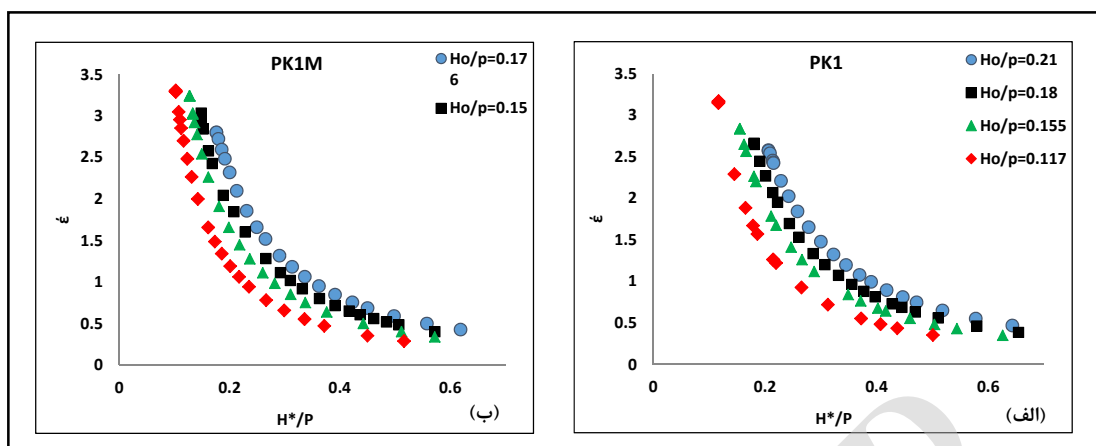
شکل ۹- منحنی تغییرات \epsilon نسبت به H^*/H_0
