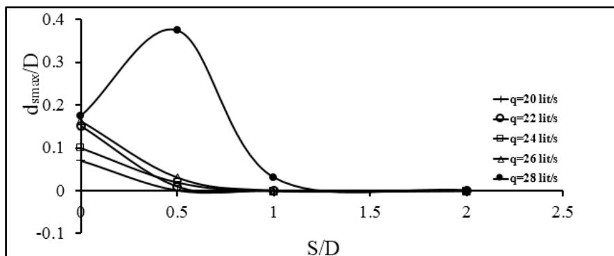
شکل ۹- حداکثر عمق آبشستگی لوله دوم در فاصله‌های مختلف
