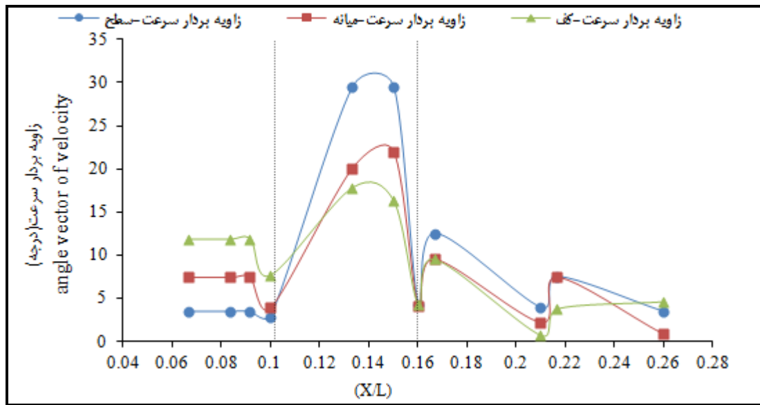
شکل ۹- تغییرات زاویه بردار سرعت در جلو دهانه آبگیر در حالت وجود سازه دیوار جداکننده و آبشکن
