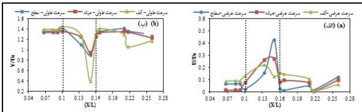
شکل ۵-الف) تغییرات سرعت طولی و ب) سرعت عرضی در جلو دهانه آبیگر در نزدیکی سطح، میانه، و بستر در حالت وجود سازه دیوار جداکننده
