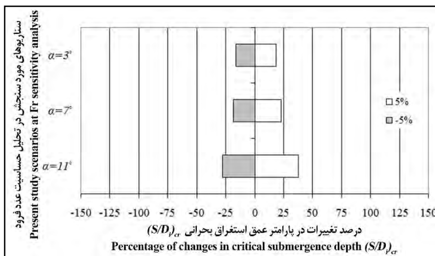
شکل ۱۲- تحلیل حساسیت پارامتر (S/Di)_{cr} برای تغییر به میزان \pm 5\% درصد در اعداد فرود مورد آزمون
