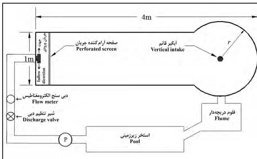
شکل ۳- پلان سیستم آزمایشگاهی Fig. 3- Experimental set-up plan
