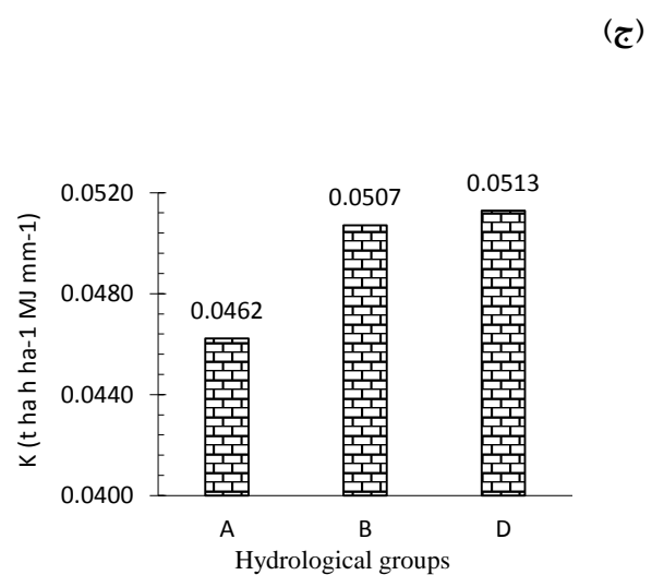
شکل ۶- مقایسه برخی ویژگی‌های زمین منظر با مقدار فرسایش‌پذیری خاک در منطقه مورد مطالعه
