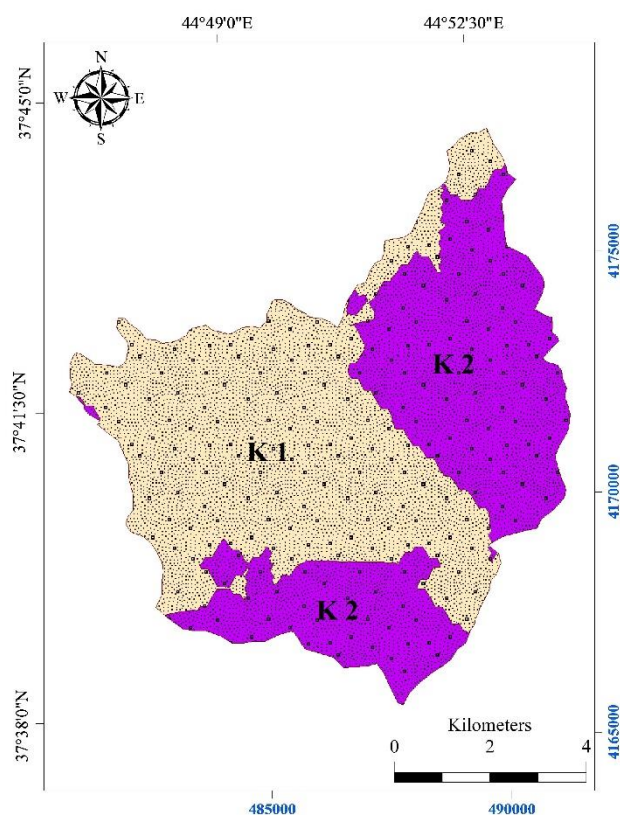
شکل ۵- پهنه بندی فرسایش پذیری خاک منطقه مورد مطالعه براساس شاخص فرسایش پذیری ویشمایر و اسمیت
