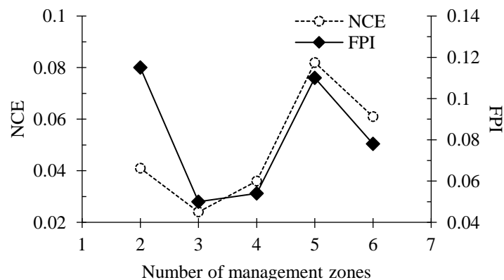
شکل ۴- آنتروپی طبقه‌بندی نرمال شده (NCE) و شاخص عملکرد فازی (FPI) محاسبه شده برای شناسایی نواحی مدیریتی بهینه
