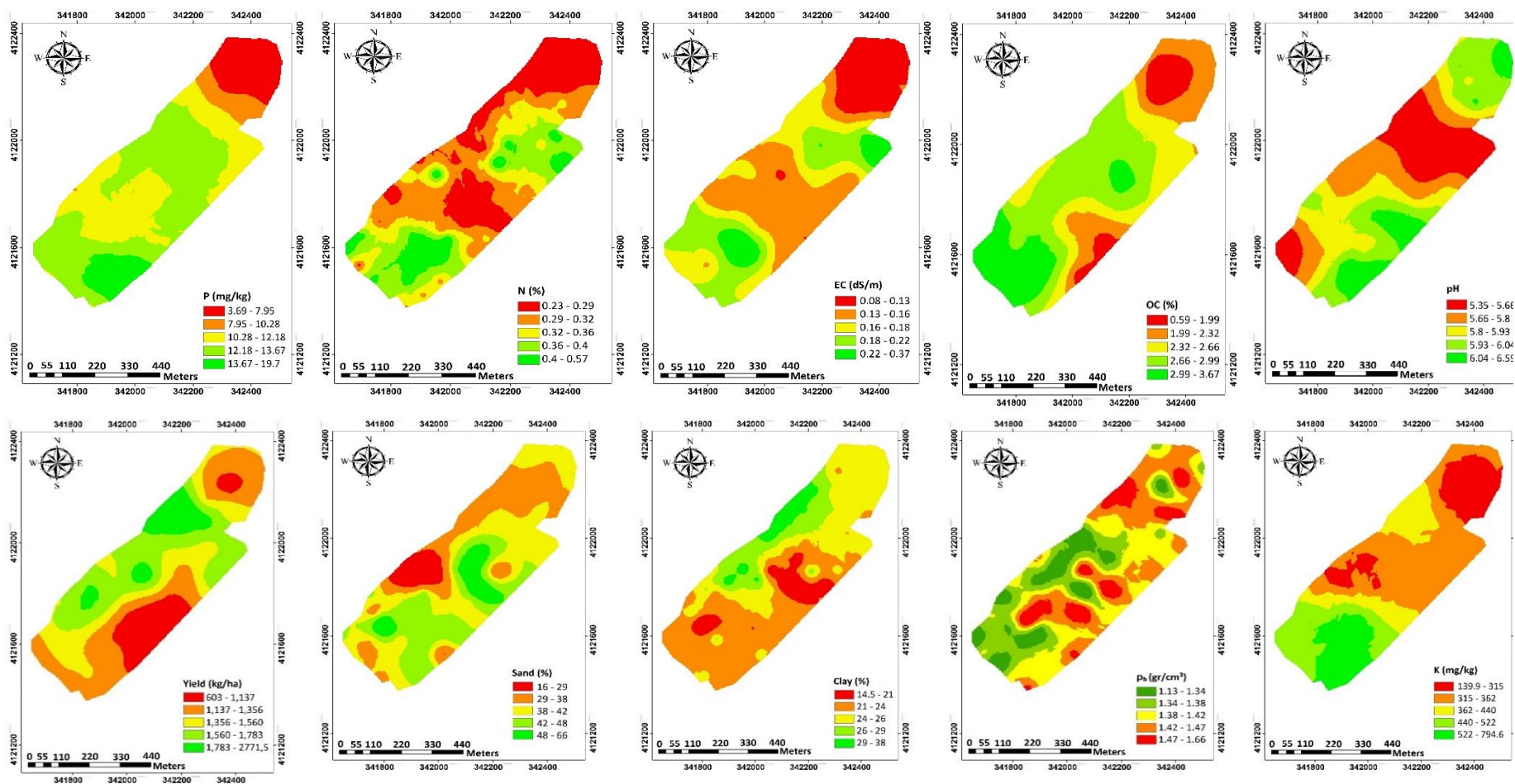
شکل ۳- توزیع مکانی ویژگی‌های خاک و عملکرد چای
