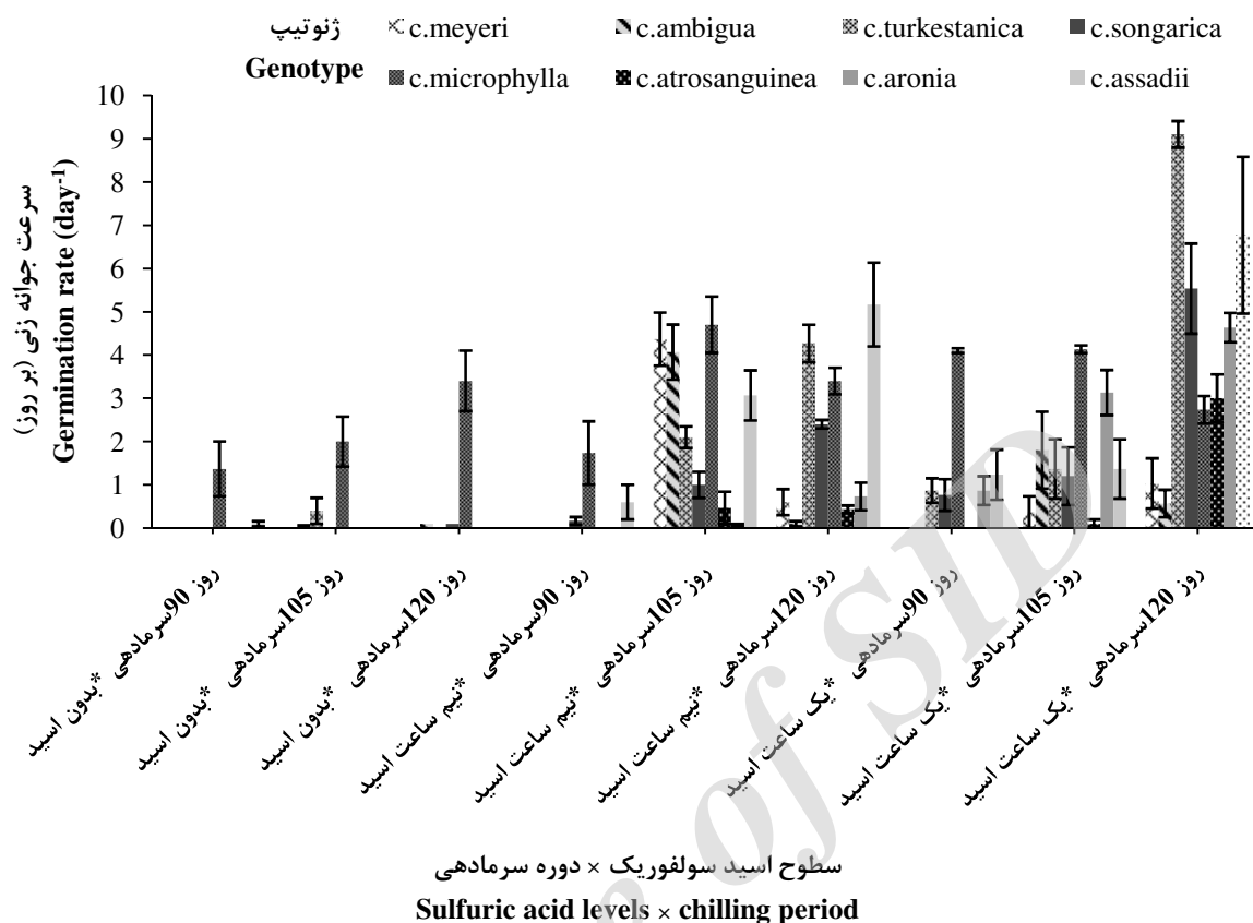
شکل ۲- برهمکنش تیمارهای اسید سولفوریک، دوره سرمادهی و ژنوتیپ برای سرعت جوانه‌زنی. بارها نشان‌دهنده خطای استاندارد میانگین‌ها می‌باشند (در ۳ تکرار)
