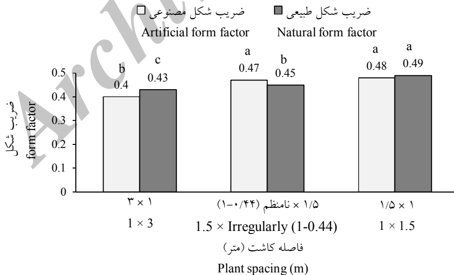
شکل ۴- میانگین ضریب شکل طبیعی و مصنوعی در سه توده با فاصله‌های کاشت متفاوت (۵ درصد \alpha=0.05 )
