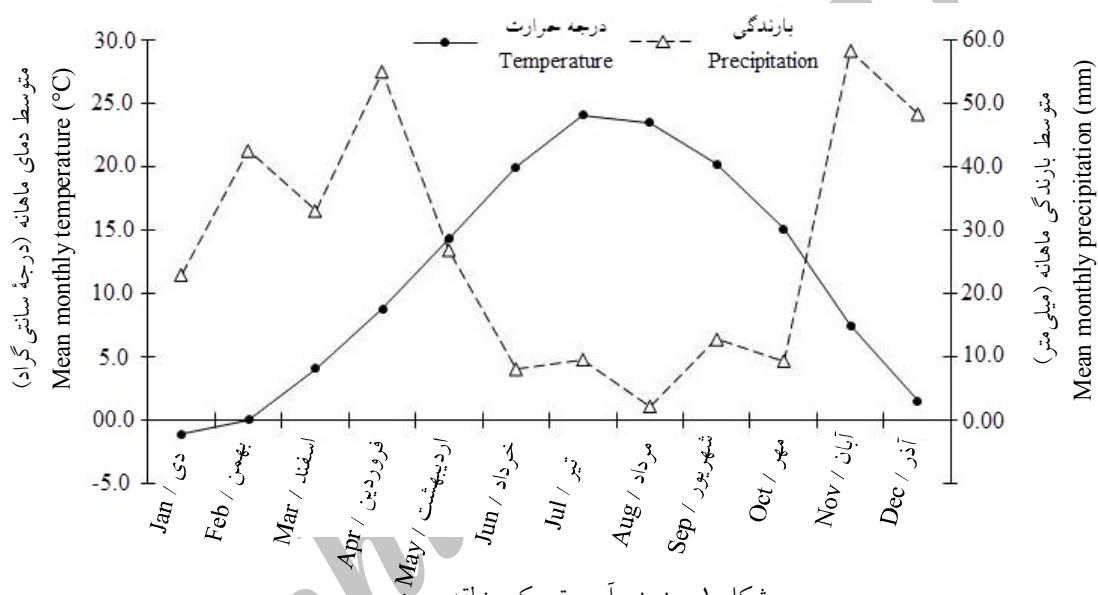
شکل ۱- منحنی آمبروترمیک منطقه مورد بررسی
