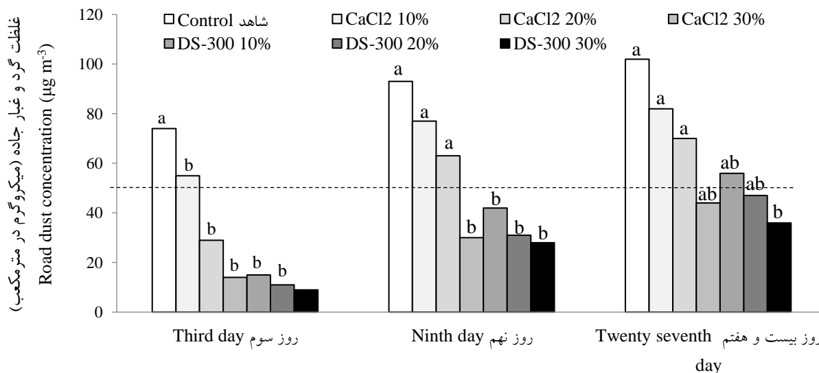
شکل ۴- وضعیت غلظت گردوغبار جاده‌ها با توجه به حد مجاز انتشار غبار (۵۰ میکروگرم در مترمکعب)
