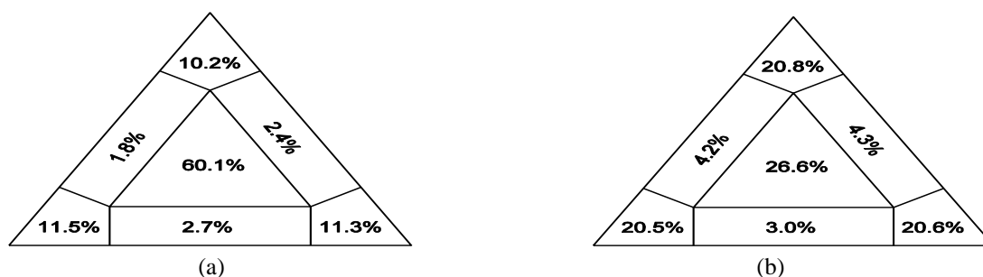
شکل ۱- (a): آنالیز LMA مربوط به داده‌های ناحیه ITS1-5.8s rDNA-ITS2، (b): آنالیز LMA مربوط به داده‌های ناحیه trnL ژن کلروپلاستی
