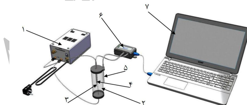
شکل ۱: دستگاه منبع حرارت خطی
