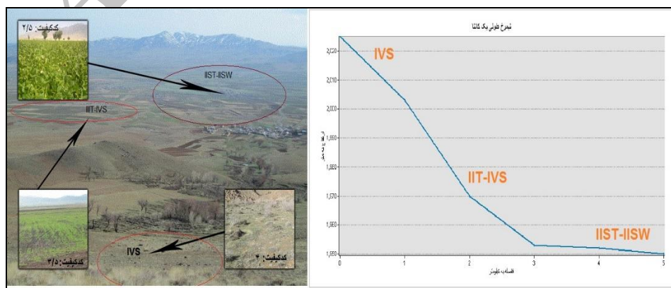
شکل ۵- اراضی متفاوت در نیم‌رخ یک شیب، IVS: خاک‌های روی دامنه و اراضی با کد کیفیت ۴، IIVS: خاک‌های با توپوگرافی ملایم و کد کیفیت ۳/۵، IISW: اراضی هموار و شیب بسیار کم با کد کیفیت ۲/۵. شیب رابطه‌ای مستقیم با کیفیت خاک دارد
