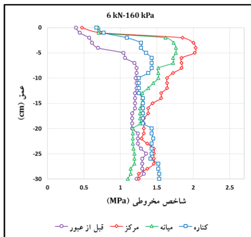
شکل ۸- تغییرات مقاومت به نفوذ، قبل و بعد از عبور در سه ناحیه مرکز، میانہ و کناره رد اثر لاستیک
