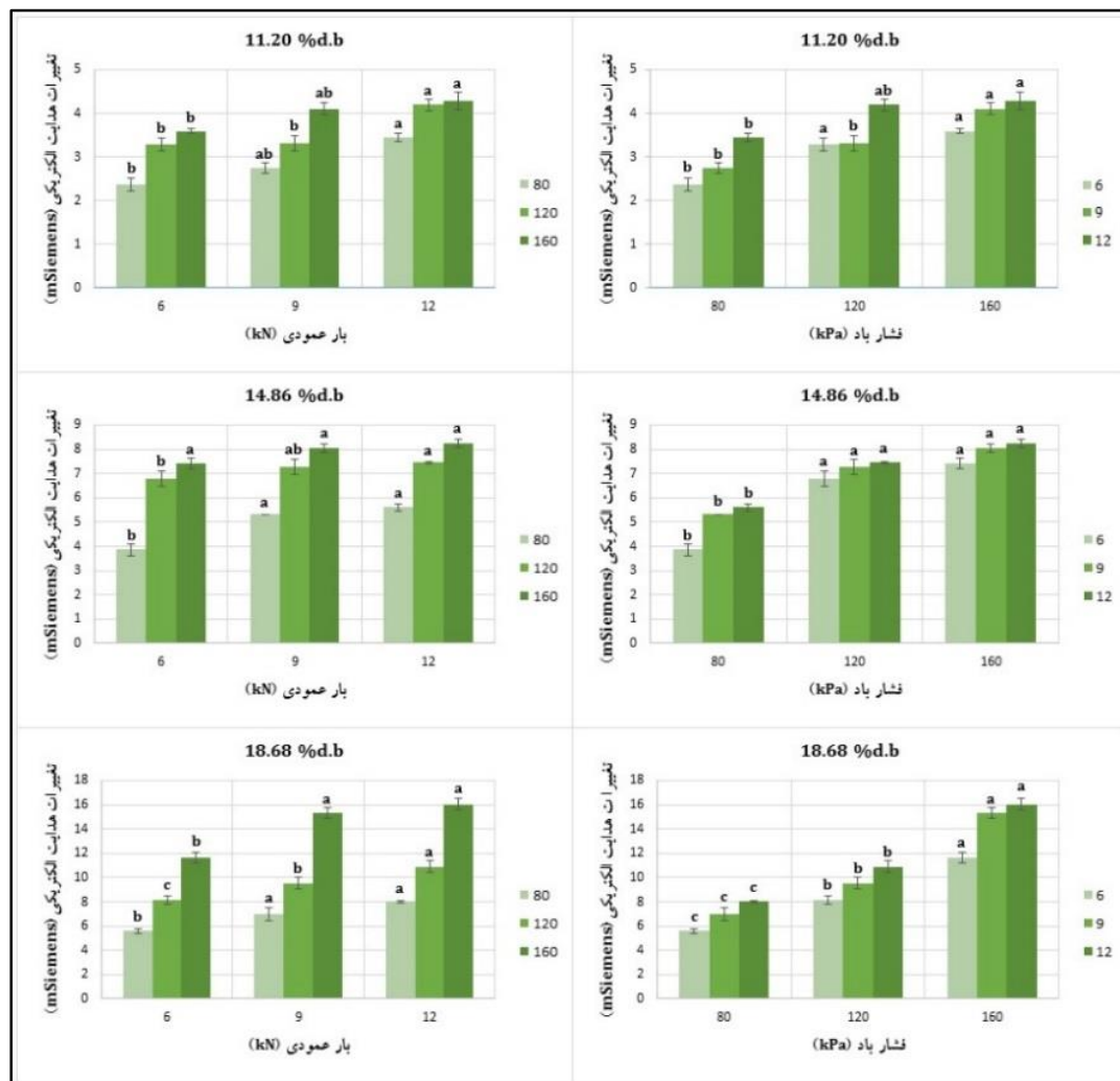
شکل ۹- تغییرات هدایت الکتریکی خاک با توجه به سطوح بار عمودی و باد لاستیک در سه سطح رطوبتی (نوار خطای بالای هر ستون نشان دهنده خطای استاندارد است)
