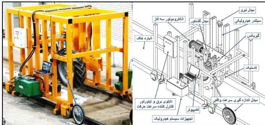
شکل ۱- سامانه آزمونگر موجود در AERI (چپ)؛ نمای شماتیکی سامانه همراه با اجزای آن (راست)
