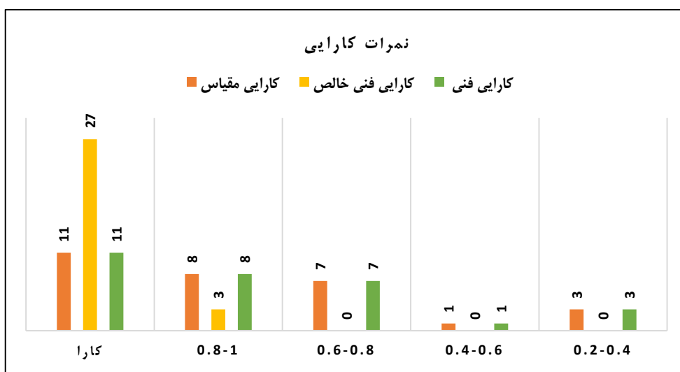
شکل ۱- فراوانی واحدها از نظر امتیاز کارایی در مصرف انرژی کلوچه
