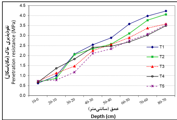
شکل ۱- تأثیر روش‌های خاک‌ورزی-کاشت بر میزان نفوذپذیری خاک Fig. 1-Effect of tillage-planting methods on soil penetration resistance
