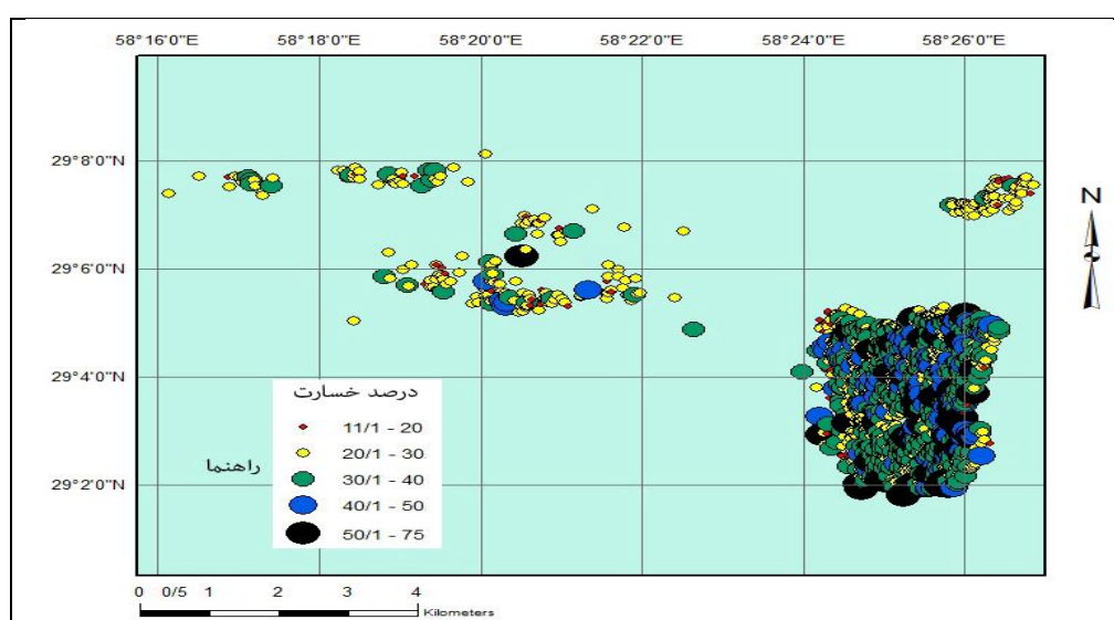
شکل ۳- نقشه پراکنش و شدت خسارت به باغ‌هایی که عارضه خشکیدگی خوشه خرما در آنها گزارش شده است. Figure 5- Distribution and severity map of orchards in which drying blossom of date palm has been reported
