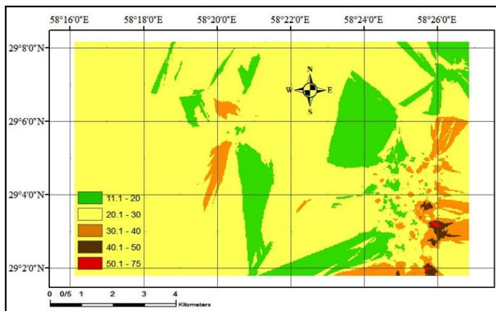
شکل ۶- نقشه سطحی شدت خسارت عارضه خشکیدگی خوشه خرما (روش کریجینگ) Figure 8- Drying blossom of date palm distribution and severity surface map (Kriging method)
