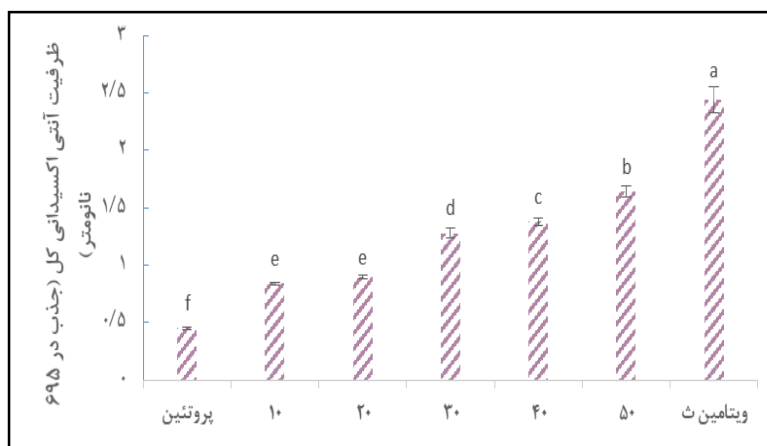
شکل ۸- مقایسه ظرفیت آنتی‌اکسیدانی کل پروتئین هیدرولیز شده در غلظت ۱۰-۵۰ (میلی‌گرم بر میلی‌لیتر) در برابر پروتئین اولیه ۵۰ (میلی‌گرم بر میلی‌لیتر) و ویتامین ث ۵۰ (میلی‌گرم بر میلی‌لیتر)
