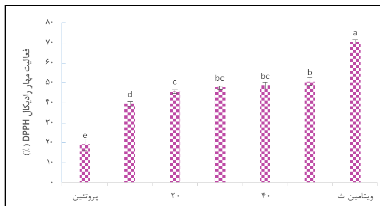
شکل ۷- مقایسه فعالیت مهار رادیکال DPPH با پروتئین هیدرولیز شده در غلظت ۱۰-۵۰ (میلی گرم بر میلی لیتر) در برابر پروتئین اولیه ۵۰ (میلی گرم بر میلی لیتر) و ویتامین ث ۵۰ (میلی گرم بر میلی لیتر)
