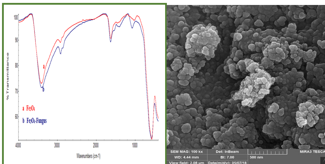
شکل ۱- تصویر میکروسکوپ الکترونی روبشی \text{Fe}_3\text{O}_4@fungus (راست) و طیف‌سنجی مادون قرمز \text{Fe}_3\text{O}_4 (a) و \text{Fe}_3\text{O}_4@fungus (b) (چپ)
