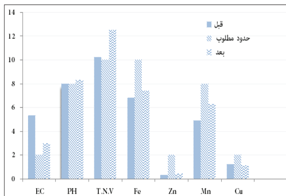
شکل ۳- مشخصات فیزیکی و شیمیایی خاک مورد استفاده در پایلوت در عمق ۳۰ سانتی متری قبل و بعد از احداث (حد مطلوب براساس استاندارد سازمان حفاظت محیط زیست ۱۳۸۲)
