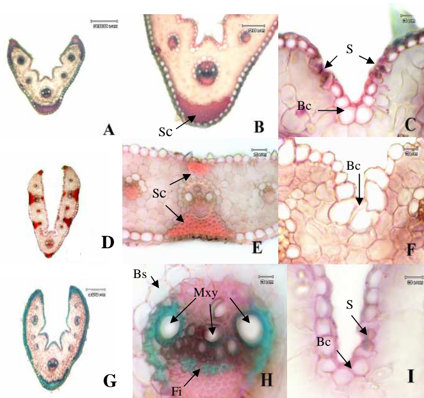
شکل ۳- مقطع عرضی برگ گونه‌های جنس Festuca : A-C: F. valesiaca D-F: F. akhanii و F. elwendiana G-I
