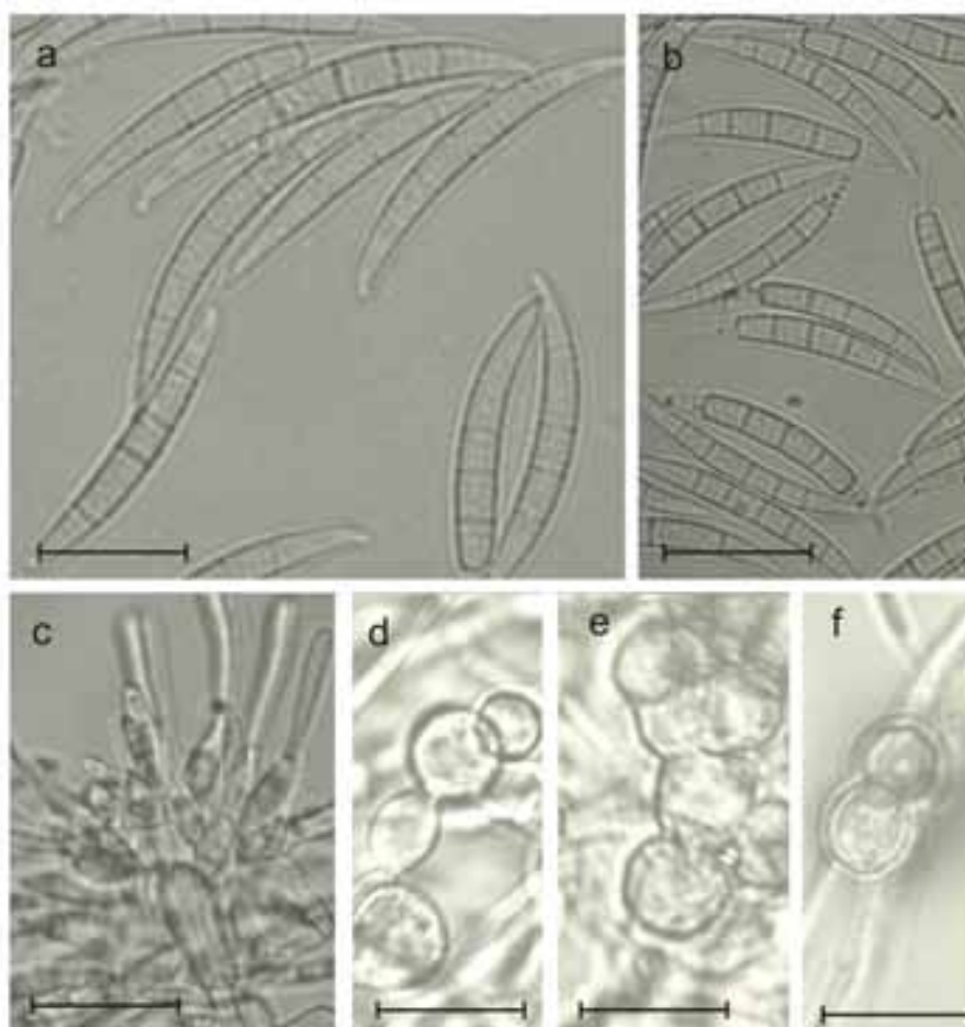
شکل ۱- Fusarium heterosporum : a-b. ماکروکنیدیوم، c. مونوفیالید منشعب، d-f. کلامیدوسپور (مقیاس برابر ۱۰ میکرومتر).
