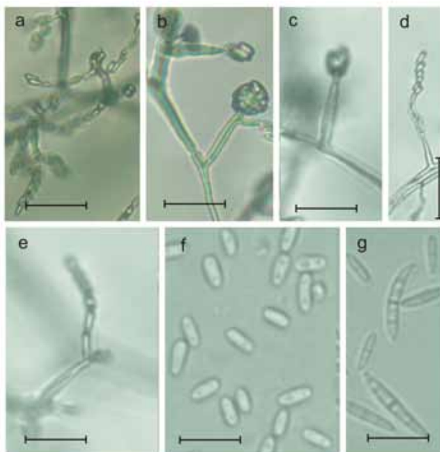
شکل ۳- Fusarium pseudonygamai : a, d, e. زنجیر کنیدیوم، b. پلی‌فیالید، c. مونوفیالید و سردروغین، f. میکروکنیدیوم، g. ماکروکنیدیوم (مقیاس a, b, d, e و برابر ۲۰ میکرومتر و c, f و برابر ۱۰ میکرومتر).
