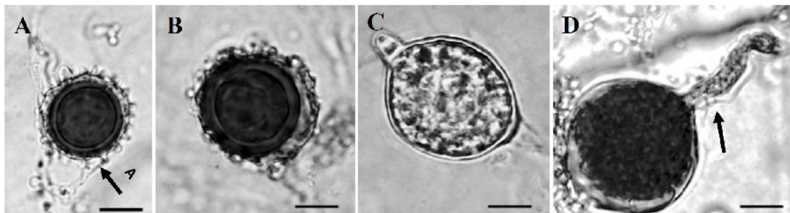
شکل ۲- ریخت‌شناسی Pythium megalacantum (جدایه MpCi03) جدا شده از شهرستان شیراز: A-B. ساختارهای جنسی: A. آسپور ناپرساز با آنتریدیوم تک‌بن، B. آسپور کاملاً ناپرساز با آنتریدیوم با اتصال پهن، C-D. اسپورانژیوم: C. اسپورانژیوم با پستانک و افزولش داخلی، D. اسپورانژیوم تقریباً تخم‌مرغی با لوله تخلیه بلند (مقیاس = ۱۰ میکرومتر).
