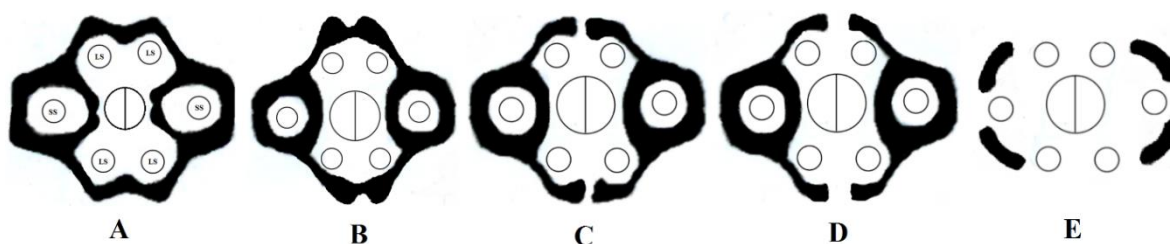
شکل ۱- تصاویر شماتیک از برش عرضی انواع نوشجای در جنس Matthiola : SS: پرچم کوتاه، LS: پرچم میانی (ترسیم توسط زراعتکار).
