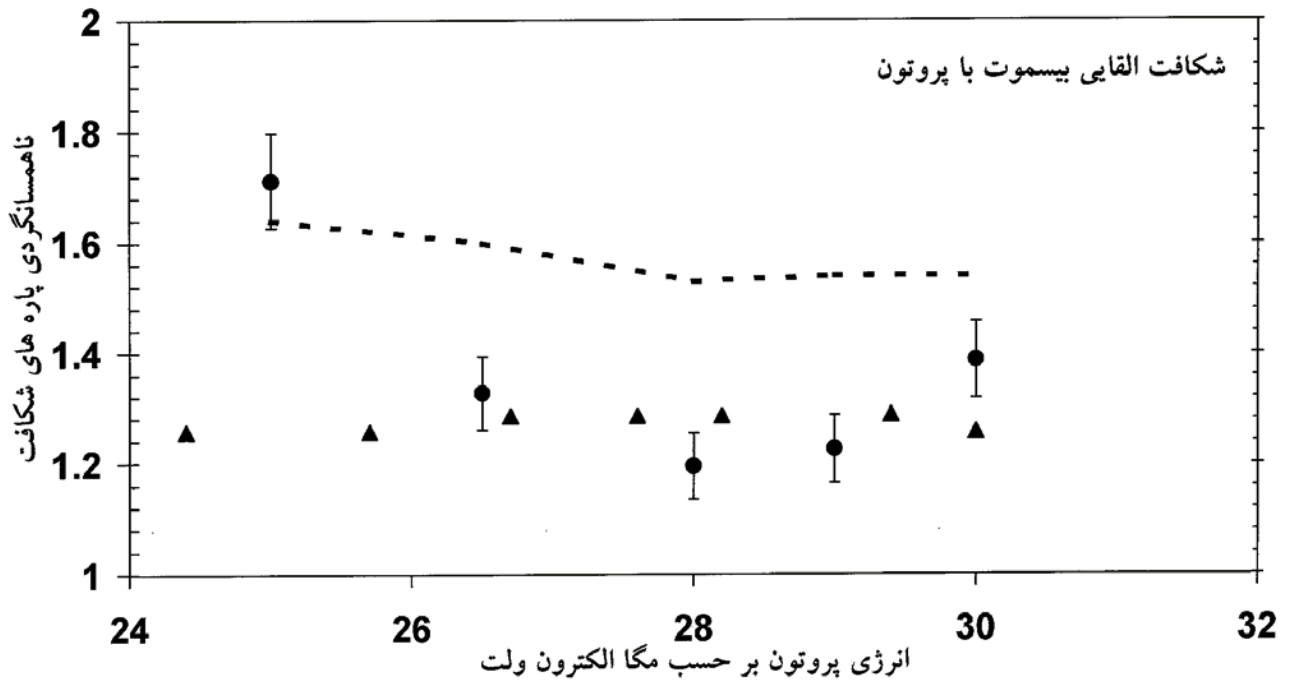
شکل ۱۵. ناهمسانگردی زاویه‌ای پاره‌های شکافت عنصر بیسموت با باریکه پروتون در انرژیهای مختلف. \Delta مربوط به مراجع [۳ و ۴]، منحنی خط چین پیش بینی مدل آماری نقطه زینی استاندارد (بدون در نظر گرفتن اسپین هسته هدف)، و \bullet مربوط به مقادیر اندازه‌گیری شده کنونی است.
