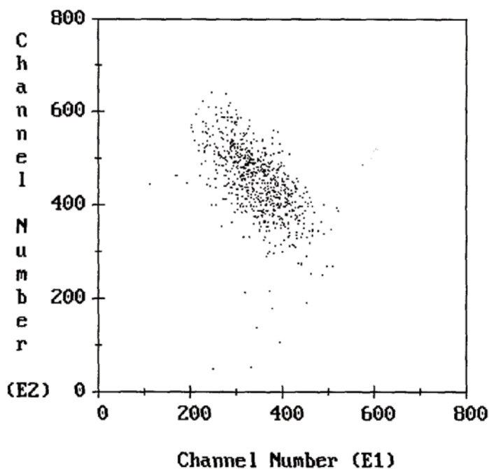
شکل ۷. توزیع دو پارامتری (شماره کانال انرژی دو پاره شکافت همفرد) در واکنش طلا با پروتونهای ۳۰ MeV آشکارساز ۲ در زاویه ۹۰ درجه نسبت به راستای باریکه تابشی قرار گرفت.
