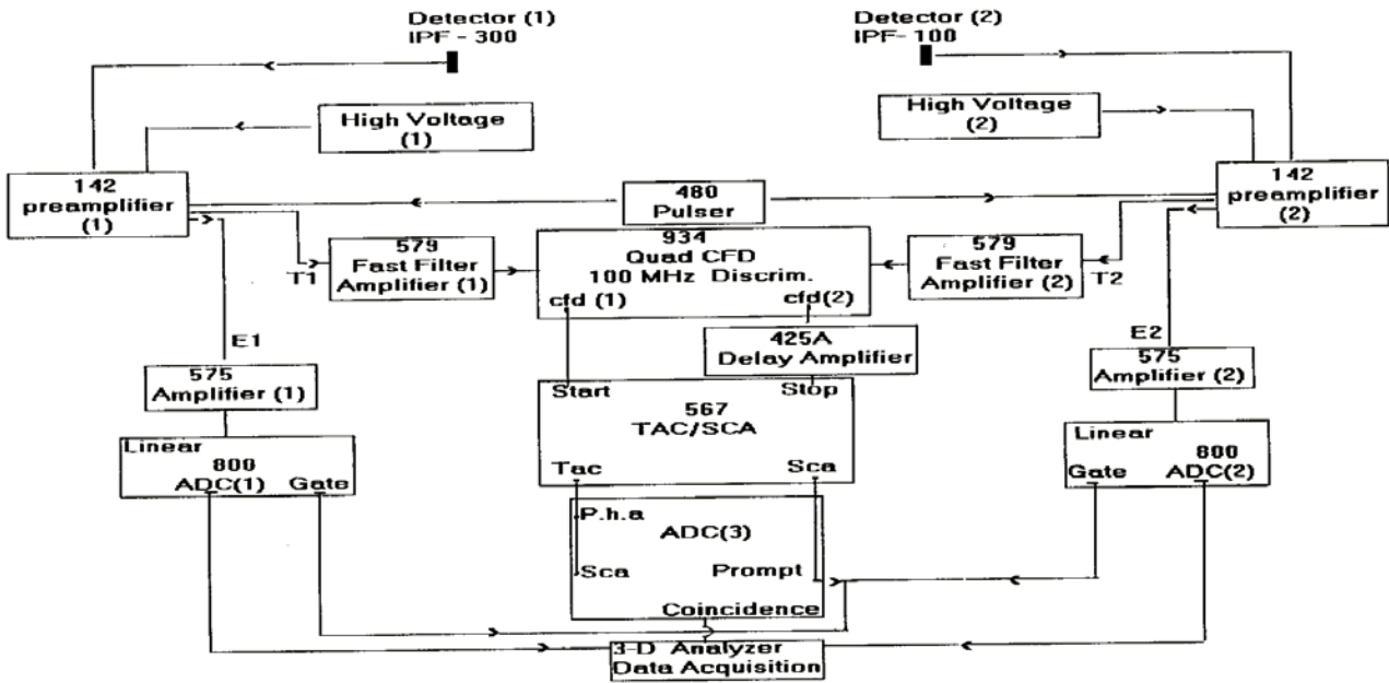
شکل ۱. مدار الکترونیک آزمایش. آشکارسازها ساخت شرکت اورسیس، ADC3 ساخت شرکت اینتر تکنیک و بقیه مدولهای الکترونیک ساخت شرکت اورتک (ORTEC) است. دستگاه جمع‌آوری داده‌ها در سازمان انرژی اتمی ایران طراحی و ساخته شده است.
