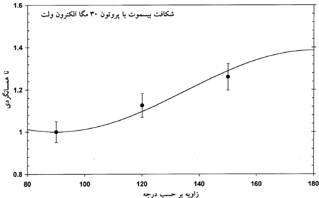
شکل ۱۳. توزیع زاویه‌ای پاره‌های شکافت عنصر بیسموت باریکه پروتون ۳۰ MeV. منحنی پربرازش با چند جمله‌ای لژاندر است.
