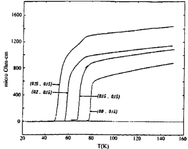
شکل ۳. منحنی مقاومت ویژه برحسب دما نمونه‌های GdPrCa-123 با غلظت ثابت یون Ca (۱۵٪) و با مقادیر متفاوت یون Pr 0/25 ، x=0/0 ، 0/15 ، 0/2 .
