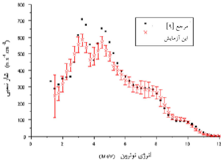
شکل ۴. مقایسه طیف Am-Be به دست آمده در این آزمایش و آزمایش کوهی و همکاران [۹] که هر دو طیف با FORIST بازیافت شده‌اند.
