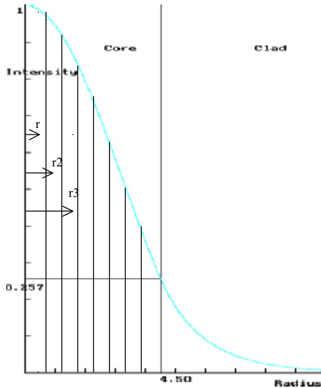
شکل ۲. پوش توان مد LP 01 پمپ در طول موج ۱/۴۸ میکرومتر در فیبر رایج تک مدی (SMF) به قسمتهایی که شدت در آنها تقریباً ثابت است، تقسیم شده است.
