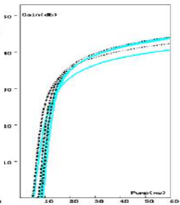
شکل ۹. منحنی بهره تقویت به توان پمپ برای فیبر با پاشندگی انتقال یافته در طول موج پمپ ۰/۹۸ میکرومتر و طولهای بهینه در توانهای پمپ ۱۰، ۲۰ و ۳۰ میلی وات.
