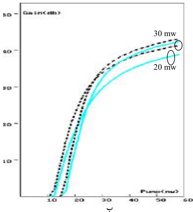
شکل ۸. منحنی بهره تقویت برحسب توان پمپ برای فیبر رایج تک مدی در طول موج پمپ ۱/۴۸ میکرومتر. شکل (الف): برای طولهای بهینه در توانهای پمپ ۱۰ و ۱۵ میلی وات و شکل (ب): بتوانهای پمپ ۲۰ و ۳۰ میلی وات.
