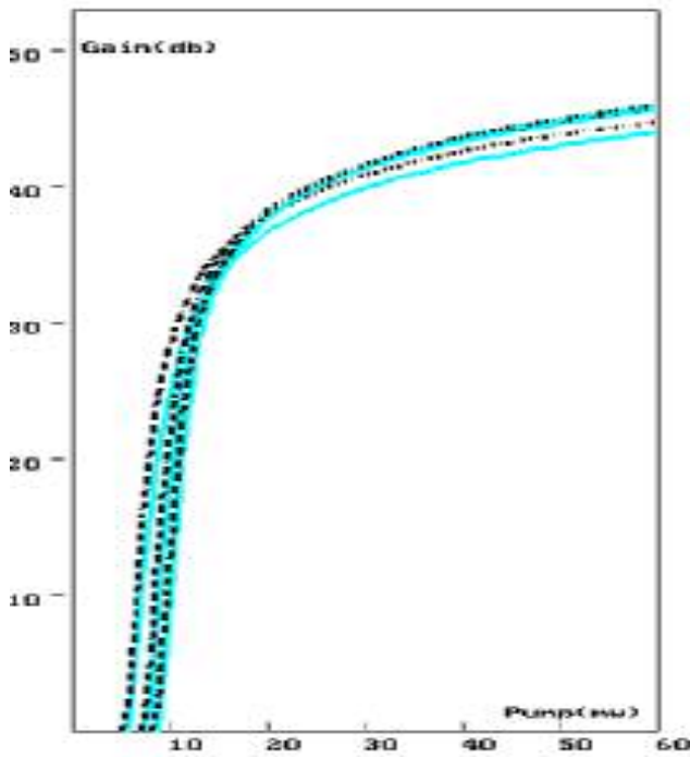
شکل ۱۰. منحنی بهره تقویت به توان پمپ برای فیبر با پاشندگی انتقال یافته در طول موج پمپ ۱/۴۸ میکرومتر و طولهای بهینه در توانهای پمپ ۱۰، ۲۰ و ۳۰ میلی وات.
