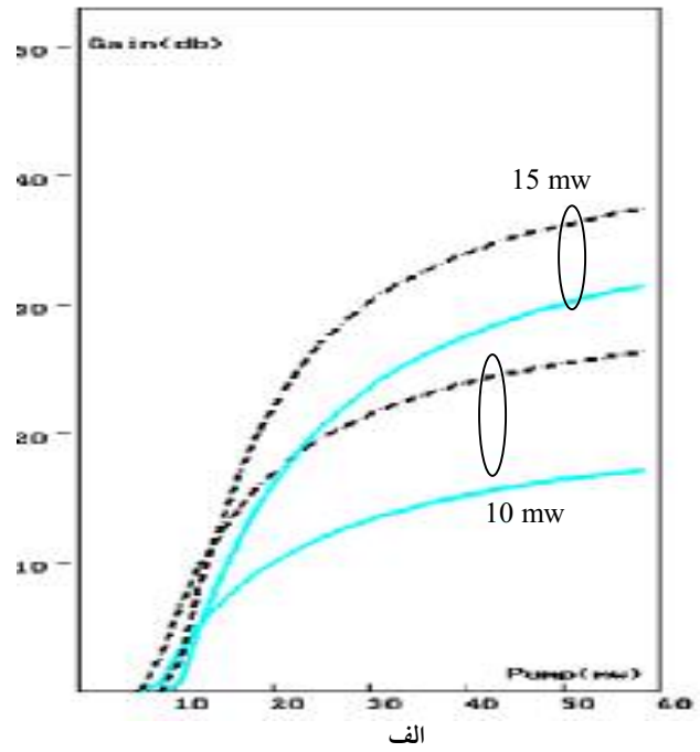
شکل ۸. منحنی بهره تقویت برحسب توان پمپ برای فیبر رایج تک مدی در طول موج پمپ ۱/۴۸ میکرومتر. شکل (الف): برای طولهای بهینه در توانهای پمپ ۱۰ و ۱۵ میلی وات و شکل (ب): بتوانهای پمپ ۲۰ و ۳۰ میلی وات.
