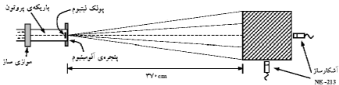
شکل ۱. هندسه آزمایش.
