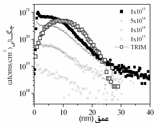
شکل ۶. نمای فسفر به دست آمده از این آزمایش برای نمونه‌هایی از فسفر کشت شده در انرژی 5 \text{ keV} ، در این شکل مقایسه‌ای با محاسبات نظری TRIM انجام شده است.
