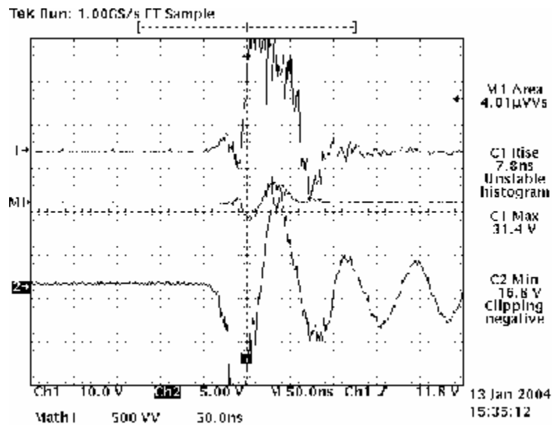
شکل ۲. رفتار جریان و ولتاژ بر حسب زمان - نوسانات ولتاژ (منحنی ۲) به دلیل وجود C_p است. قله اول در جریان (منحنی ۱) به دلیل وجود پلاسمای اولیه کرونا است. حداکثر ولتاژ اعمال شده به راکتور در نیم پریود اول حدود 17 \text{ kV} است و قله جریان اصلی پلاسما حدود 250 \text{ A} می باشد انرژی تزریق شده که با مساحت M_1 نمایش داده شده است حدود 40 \text{ mJ} است.
