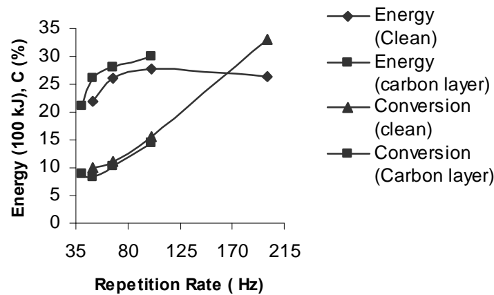
شکل ۳. بستگی تبدیل و انرژی مخصوص بر حسب فرکانس تکرار، سایر شرایط آزمایشی عبارتند از: F = 1/6 \frac{NI}{hr} (نرخ فلوی گاز)، V = 28 \text{ kV} ، C = 220 \text{ pF} .
