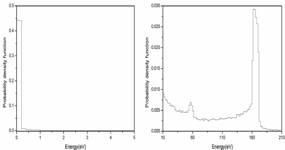
شکل ۱۳. توزیع انرژی جنبشی اتمهای میوندار در حالت پایدار مرجع [۱۰].
