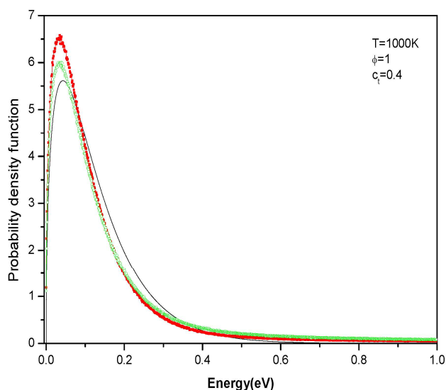
شکل ۱۵. طیف انرژی اتمهای میوندار در حالت پایدار مرجع [۱۰] در شرایط T=1000\text{K} ، \phi=1 و c_i=0.4 در لحظه t=150 \pm 1\text{ns} و مقایسه آن با توزیع انرژی اتمهای میوندار در حالت پایه ماکسولی نیست و از مرجع [۱۰] جایگزین شده باشد و مقایسه آن با توزیع انرژی اتمهای میوندار در حالت پایه ماکسولی.
