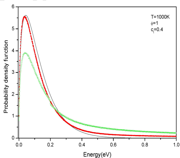
شکل ۱۴. طیف انرژی اتمهای میوندار در لحظه t\mu و t\mu' در شرایط T=1000\text{K} ، \phi=1 و c_i=0.4 در شرایطی که انرژی اولیه اتمهای میوندار در حالت پایه ماکسولی نیست و از مرجع [۱۰] جایگزین شده باشد و مقایسه آن با توزیع انرژی اتمهای میوندار در حالت پایه ماکسولی.
