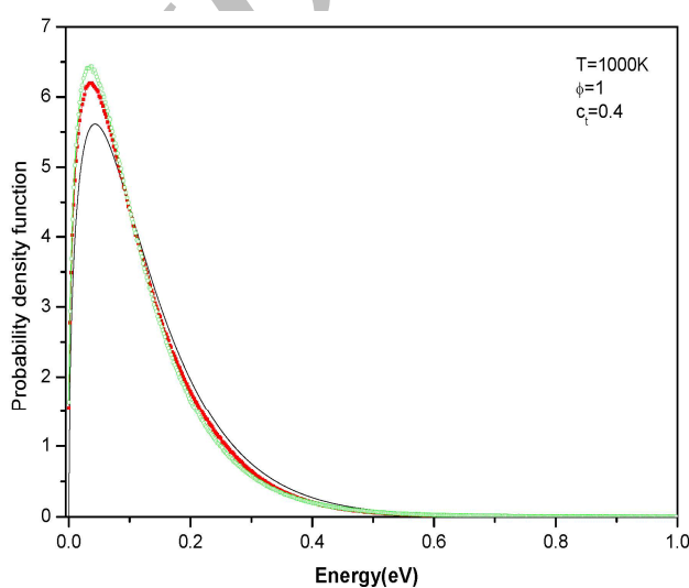
شکل ۱۱. مقایسه طیف انرژی اتمهای میوندار t\mu (■) و dt (O) در لحظه t=150 \pm 1 ns در شرایط T=1000K و \phi=1 و c_i=0.4 با توزیع انرژی ماکسولی.
