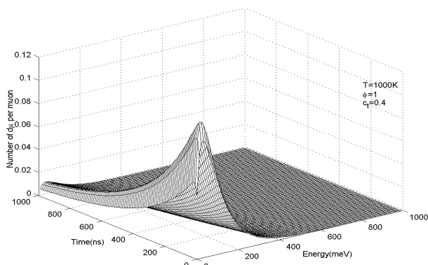
شکل ۱۰. تحول زمانی طیف انرژی اتمهای میوندار dt در شرایط T=1000K و \phi=1 و c_i=0.4 .
