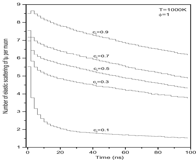
شکل ۷. طیف زمانی برخوردهای کشسان اتمهای t\mu در غلظتهای مختلف تریتیوم در شرایط T=1000K و \phi=1 .
