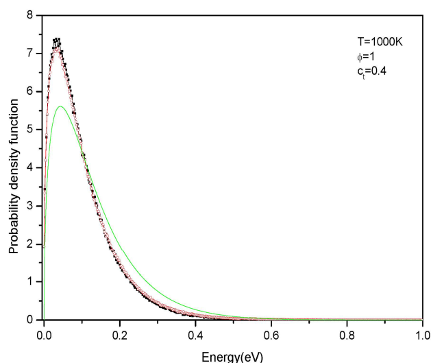
شکل ۱۲. مقایسه طیف انرژی اتمهای میوندار dt (O) و t\mu (■) در لحظه t=150 \pm 1 ns با شرایط T=1000K و \phi=1 و c_i=0.4 با توزیع انرژی ماکسولی.
