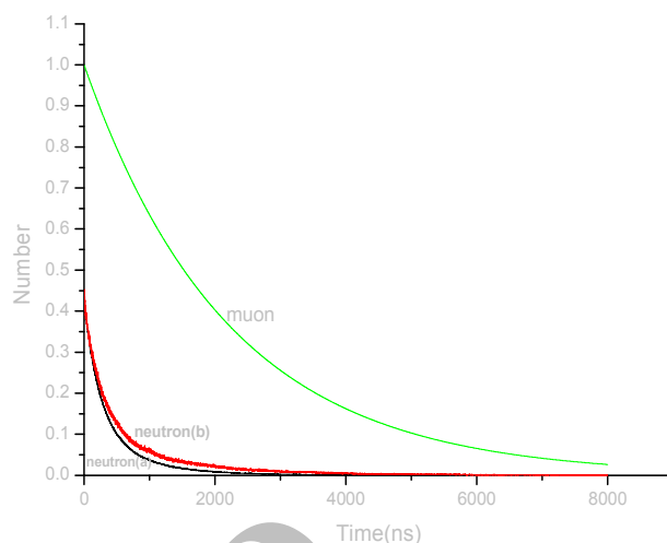
شکل ۵. طیف زمانی نوترونها همجوشی در شرایط T=1000\text{K} و \phi=1 و C_t=0.4 در دو حالت با واپاشی میون (a) و بدون آن (b) در نظر گرفتن واپاشی میون (b) و مقایسه آنها با نمودار واپاشی میون.
