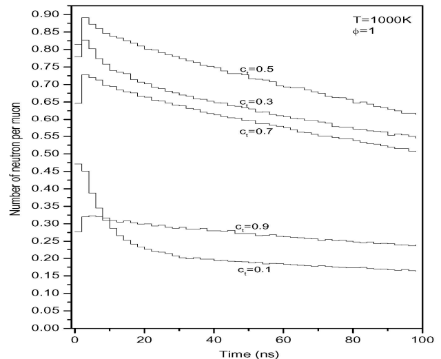
شکل ۶. طیف زمانی نوترونیهای موجود در غلظتهای مختلف تریتیوم در شرایط T=1000K و \phi=1 .
