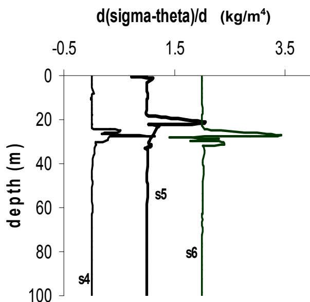
شکل ۹. الف) گرادیان قائم محلی چگالی پتانسیل برای ایستگاههای ۴ (حوضه جنوبی)، ۵ (روی پشته)، ۶ (حوضه میانی). (برای بررسی واضحتر به اندازه‌های ایستگاه ۵ یک واحد و ایستگاه ۶ دو واحد اضافه شده است).
