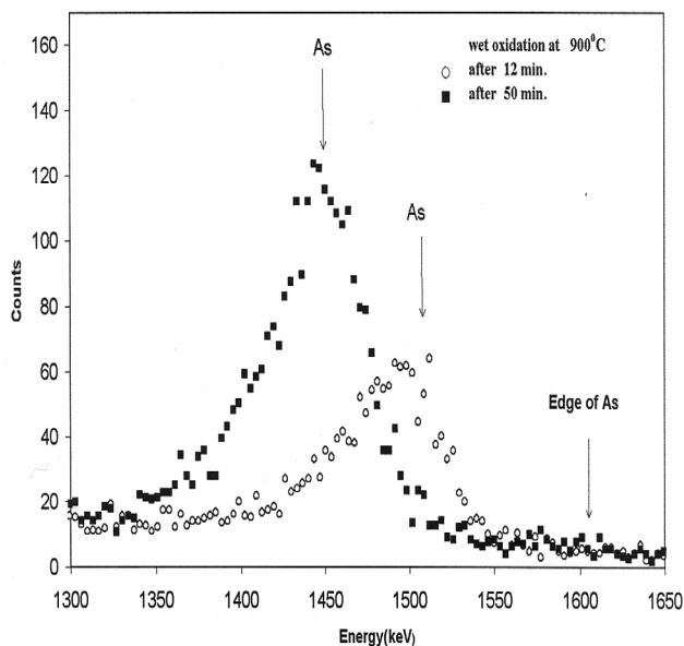
شکل ۳. تغییرات پروفایل آرسنیک در حین اکسیداسیون و در زمانهای مختلف. همان طور که مشاهده می شود با افزایش زمان اکسیداسیون، قله آرسنیک تیزتر می گردد.
