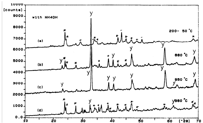
شکل ۱. طیفهای اشعه X نمونه ۱ بعد از حرارت‌دهی تا 980^{\circ}\text{C} : (d) ، 950^{\circ}\text{C} : (c) ، 880^{\circ}\text{C} : (b) ، 250-200^{\circ}\text{C} : (a) BaCO_3 (*), Y_2O_3 (+), CuO (·), YBaCuO_5 (o), YBa_2Cu_3O_{7-x} (y)
