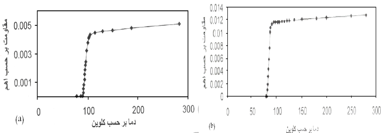
شکل ۶. نمودار تغییرات مقاومت بر حسب دما (a) نمونه ۱ و (b) نمونه ۲.
