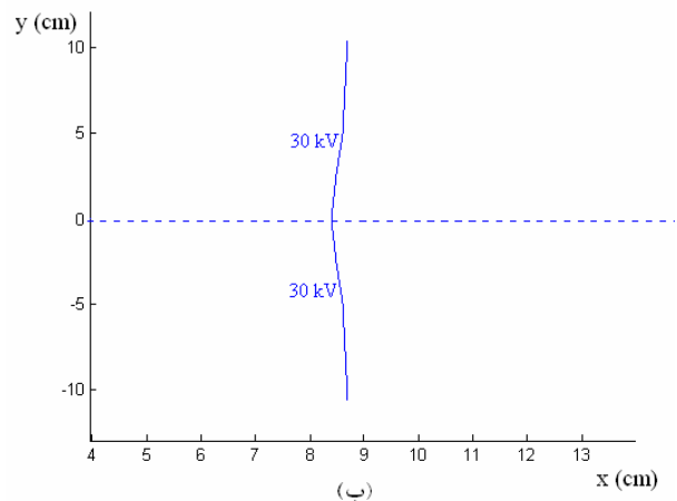
شکل ۲. سطوح هم‌پتانسیل الف) ۶۰ kV و ب) ۳۰ kV.
