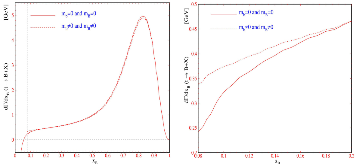
شکل ۳: اثر جرم هادرون و کوآرک bottom روی توزیع انرژی هادرون نهایی B از واپاشی کوآرک Top. پارامترهای در نظر گرفته شده عبارتند از: m_b = 4.5 \text{ GeV} , m_B = 5.28 \text{ GeV} , m_t = 174 \text{ GeV} , m_W = 80 \text{ GeV} و \mu_s = 4.5 \text{ GeV} .
