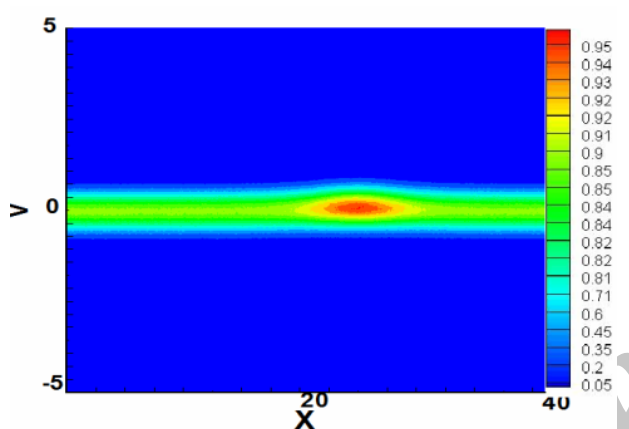
شکل ۱۷. منحنی فضای فاز یونی در زمان t=3 .
