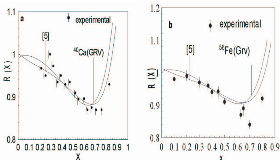
شکل ۲. در نمودار a و b نسبت R(x) = \frac{F_x^A}{F_x^D} که تابعی از x برای هسته‌های ^{40}\text{Ca} و ^{56}\text{Fe} است با در نظر گرفتن اثرات انرژی بستگی هسته‌ای محاسبه شده است و داده‌های تجربی از مرجع [۱۳] گرفته شده‌اند.
