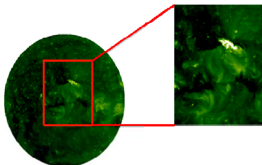
شکل ۱. تصویر قرص کامل خورشید و ناحیه پرتاب جرم تاجی از طول موج ۱۹۵ آنگستروم استرو مربوط به ۲۶ آوریل ۲۰۰۸ نمایش داده شده است.
